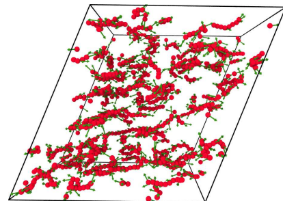
(d) \lambda = 6.17 , Shear thinning regime
