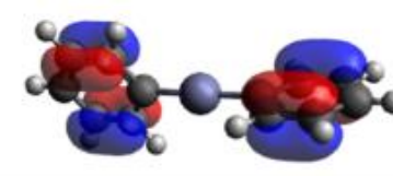
HOMO-3
