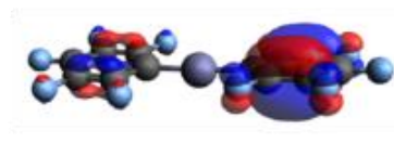
HOMO-1
