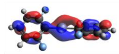
LUMO+1
