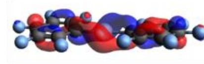
LUMO+1
