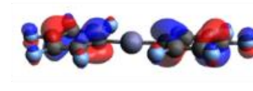
HOMO-3
