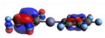
HOMO
