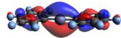
LUMO
