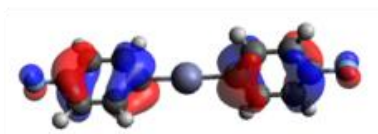
HOMO-1
